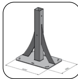
Steherfuß
