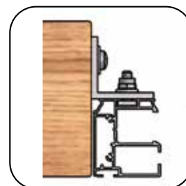
Laibungswinkel
