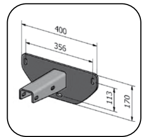
Wandkonsole (optional)
