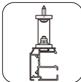
Distanzkonsole
